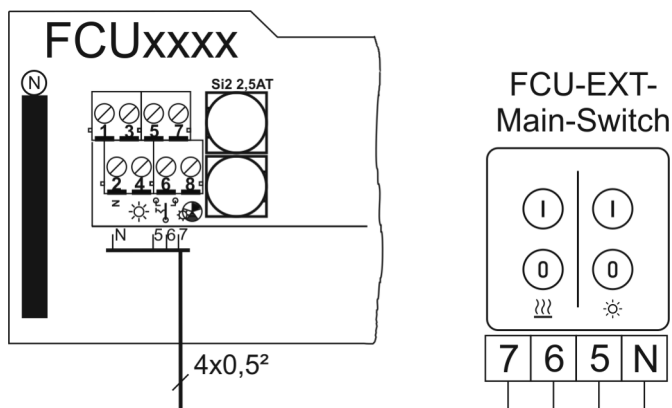
Рисунок 15: Соединение Внешний главный выключатель
