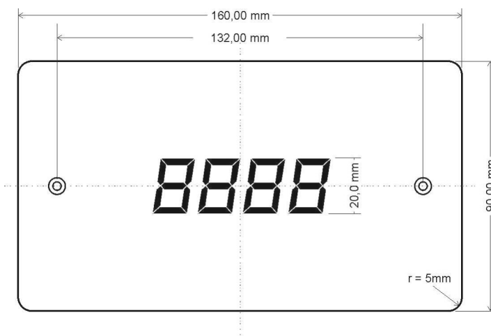
Рисунок 7: Размеры внутреннего дисплея
