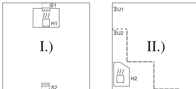
Рис 4 : Установка лавочного, печного или комбинированного типа датчиков
