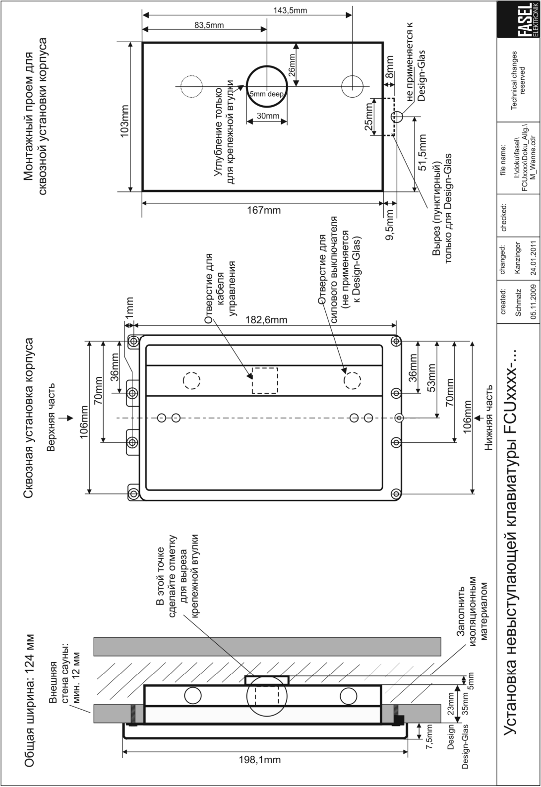
Рисунок 1: Монтажный проем для элемента управления FCUxxxx-Design и FCUxxxx-Design-Glas
