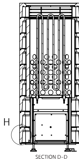
SECTION D-D
